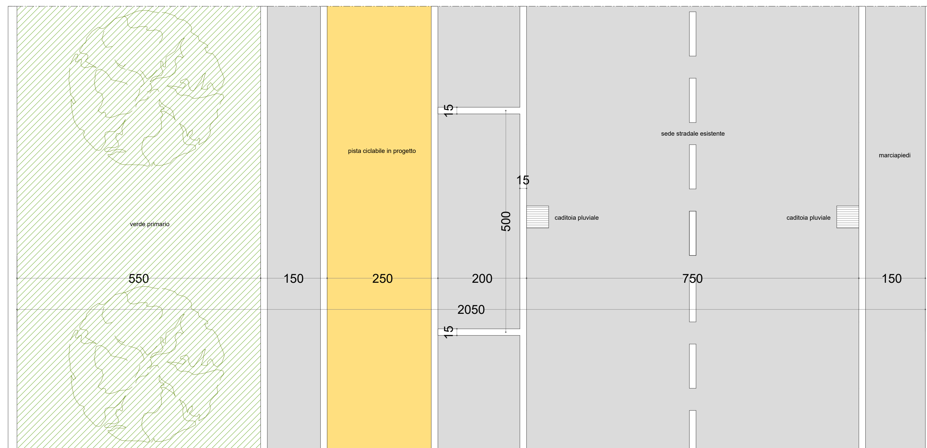
Pianta stradale tipo S1
