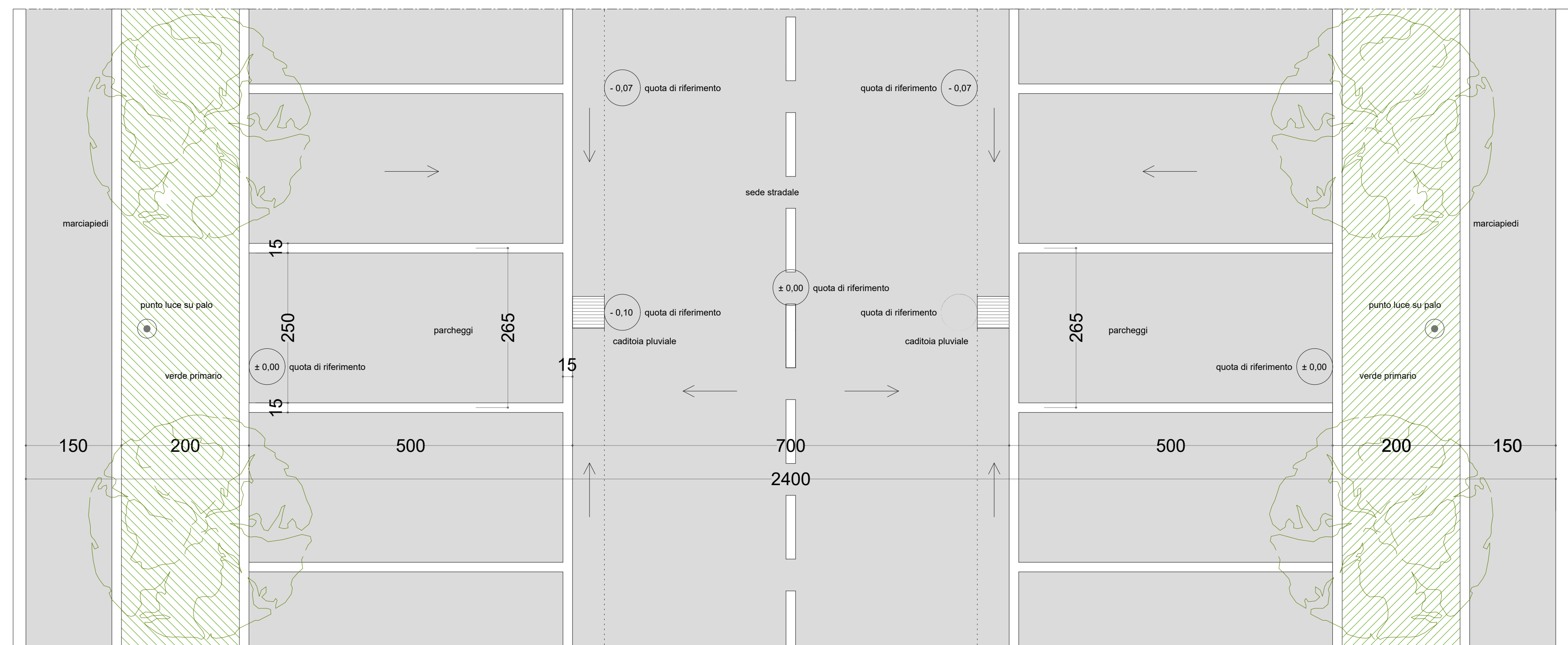
Pianta stradale tipo S2
